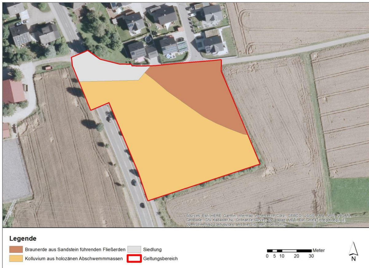
Abb. 2: Bodentypen im Geltungsbereich gem. BK 50 (Quelle Luftbild: ESRI).
